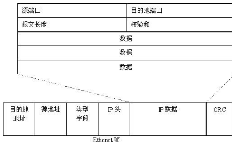
图 5-4 UDP 头
